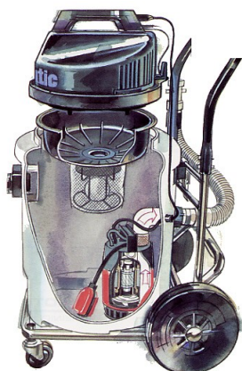
Behälter mit eingebauter Tauchpumpe
