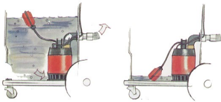
Automatische Tauchpumpe Behälter voll - Pumpe ein Behälter leer - Pumpe aus
