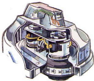
Motorkopf mit 2 Motoren
